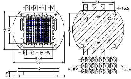
产品规格 Product dimension
