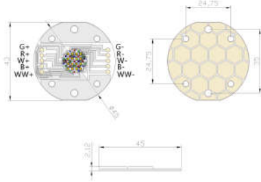
产品规格 Product dimension
