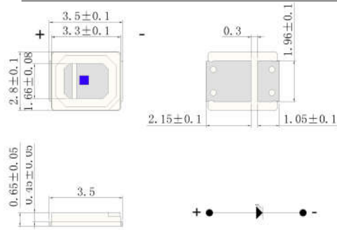
产品规格 Product dimension
