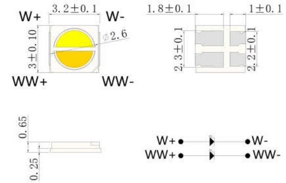
产品规格 Product dimension
