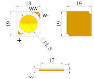
产品规格 Product dimension
