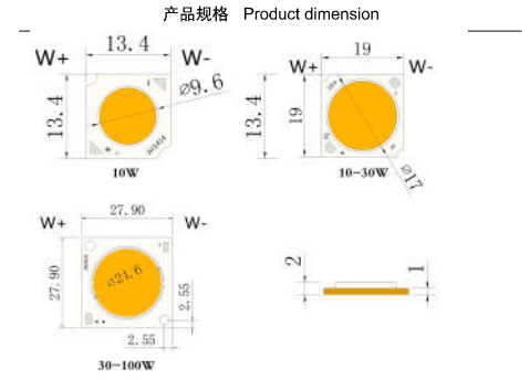
产品规格 Product dimension
