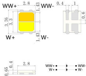
产品规格 Product dimension
