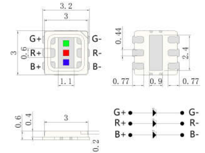
产品规格 Product dimension
